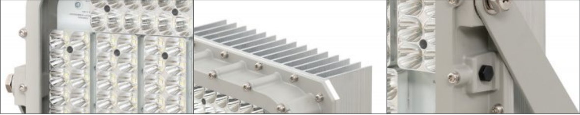
눈부심 없는 리플렉터 광학구조 수직 압출 구조로 방열효과 우수 모듈별 Air vent 적용하여 결로방지
