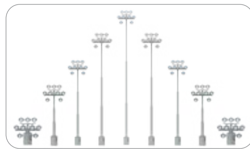
－ 다단식 조명탑 승,하강시 모습
